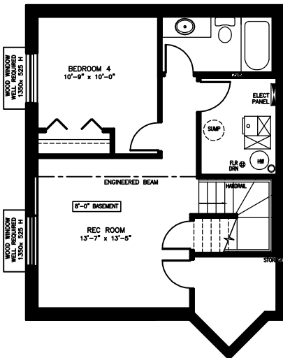
OPTIONAL BASEMENT PLAN
